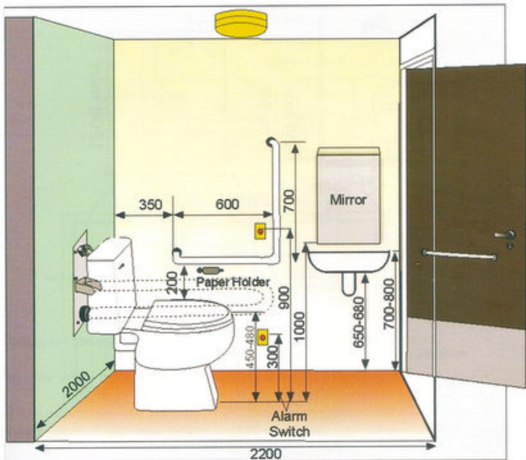
Fig. 52 Accessible Toilet
